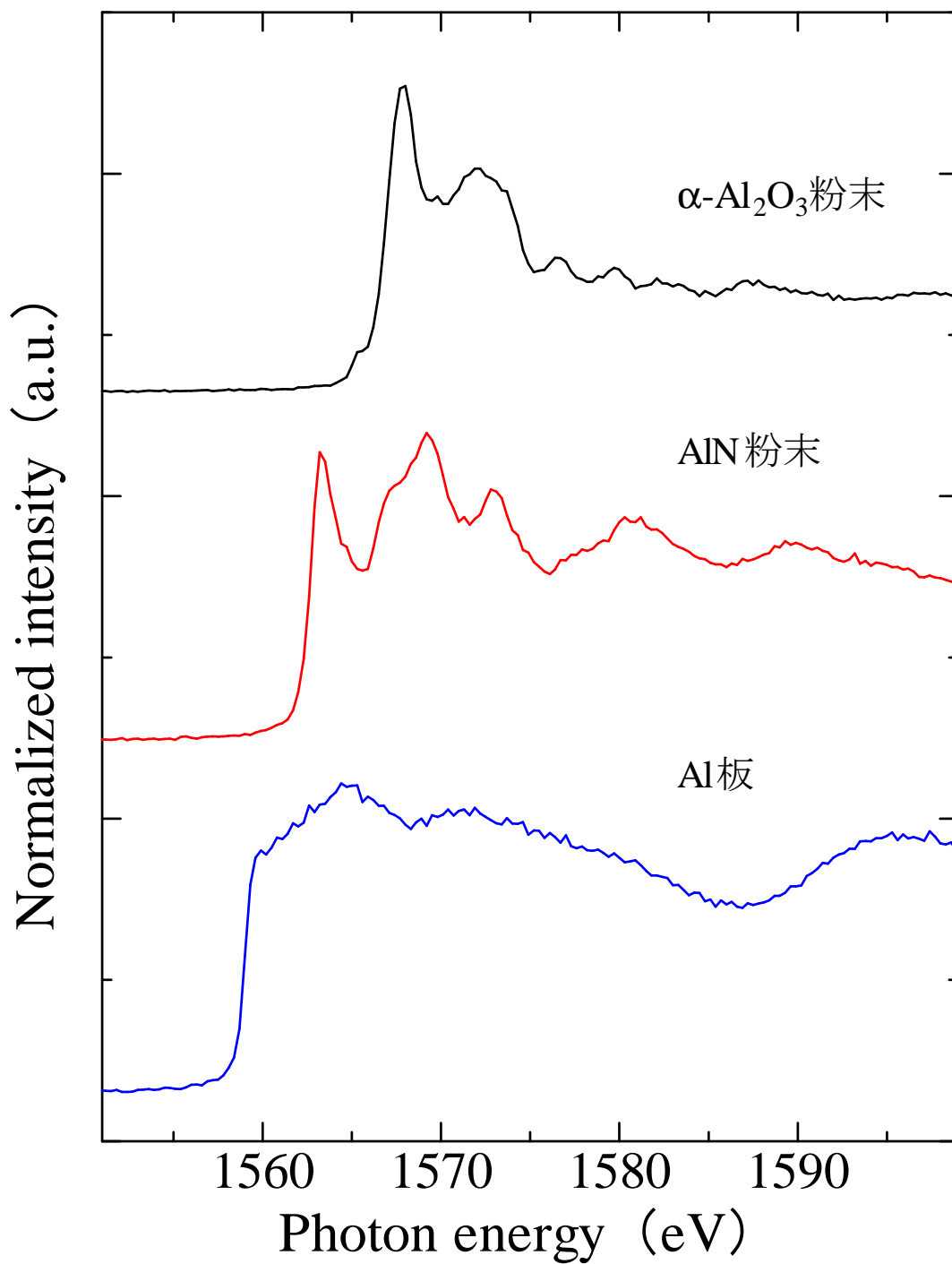
Al- K 吸収端XANESスペクトル (蛍光収量法)
