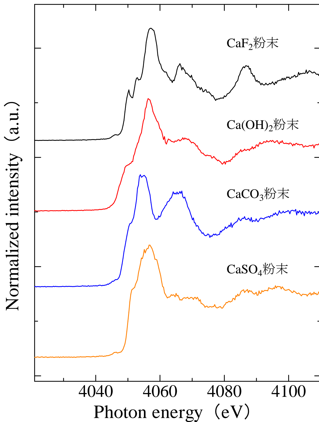
Ca- K 吸収端XANESスペクトル (蛍光収量法)
