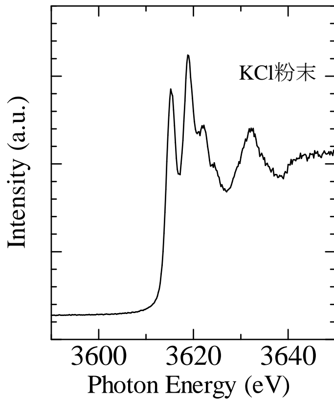
K- K 吸収端XANESスペクトル (蛍光収量法)
