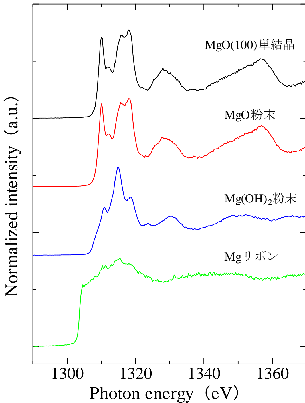
Mg- K 吸収端XANESスペクトル（蛍光収量法）
